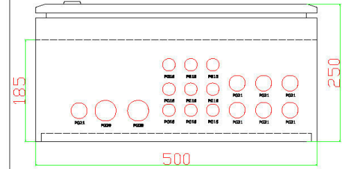
PANO ALT REKOR GİRİŞİ GÖRÜNÜŞ
