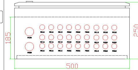
PANO ALT REKOR GİRİŞİ GÖRÜNÜŞ
