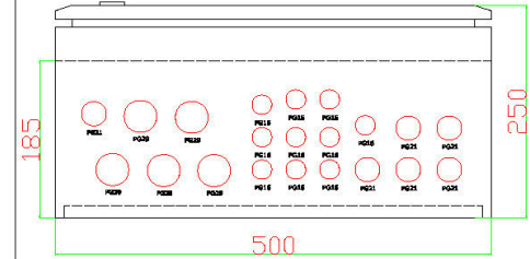
PANO ALT REKOR GİRİŞİ GÖRÜNÜŞ
