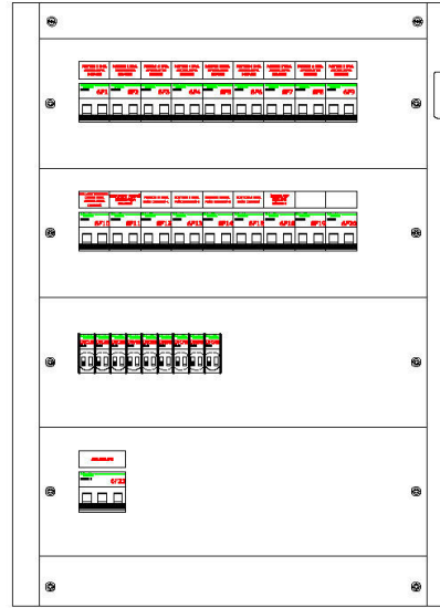
EMNİYETLİ İÇ GÖRÜNÜŞ
