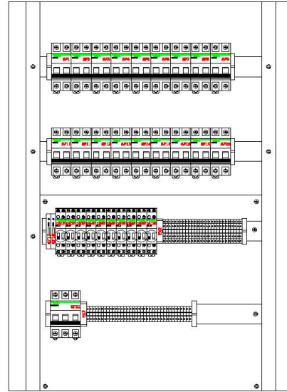
İÇ YERLEŞİM GÖRÜNÜŞ
