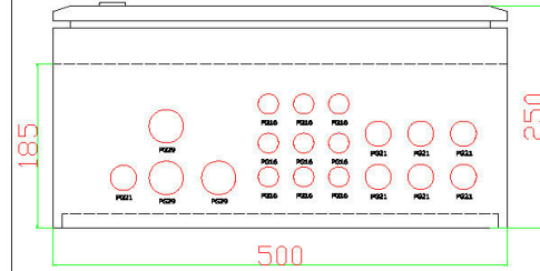
PANO ALT REKOR GİRİŞİ GÖRÜNÜŞÜ
