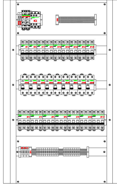
İÇ YERLEŞİM GÖRÜNÜŞÜ
